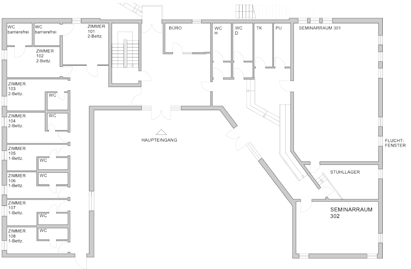
REHGARTEN GRUNDRISS ERDGESCHOSS 1:100
